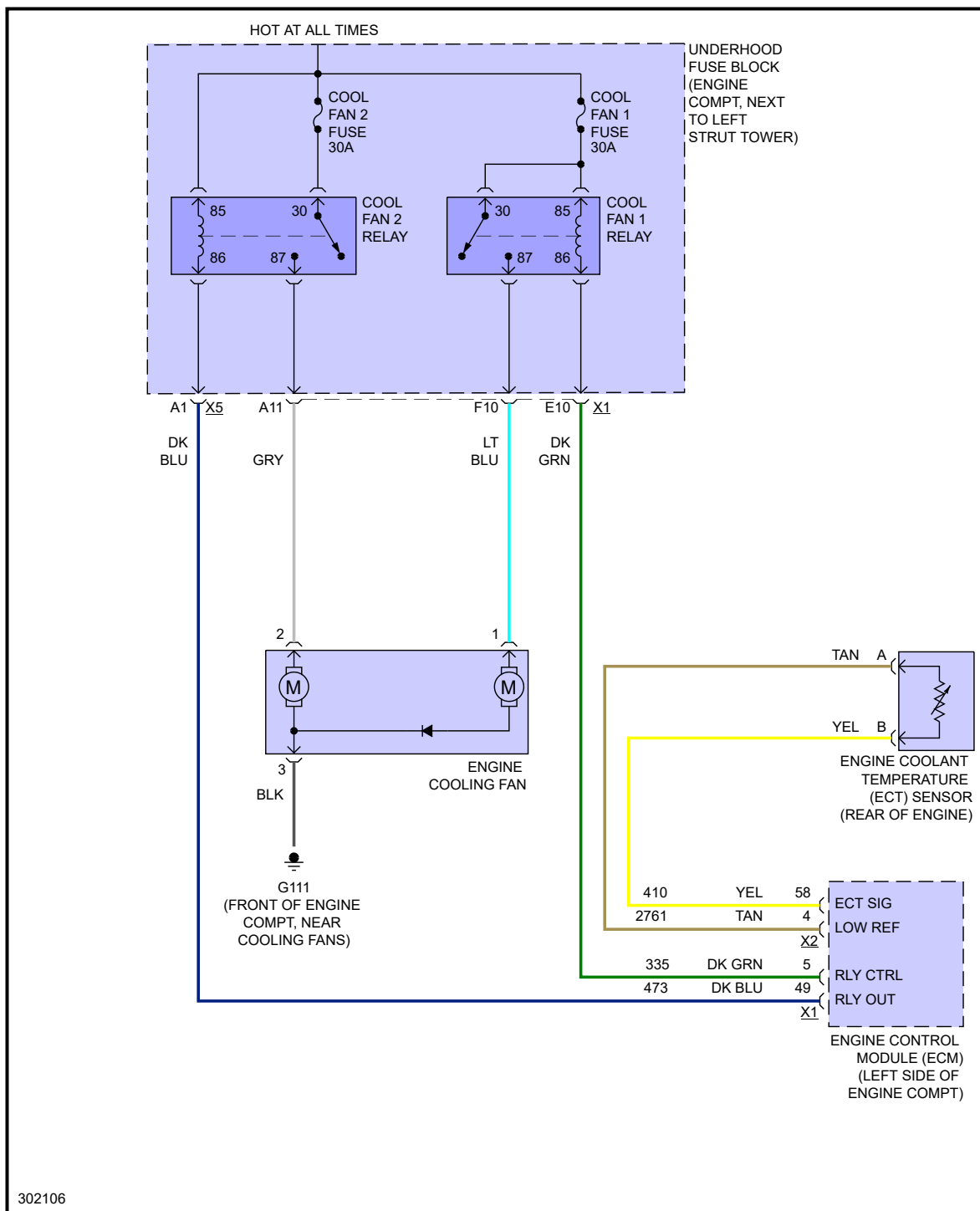
Fig 1: 2.2L VIN 5, Cooling Fan Circuit
