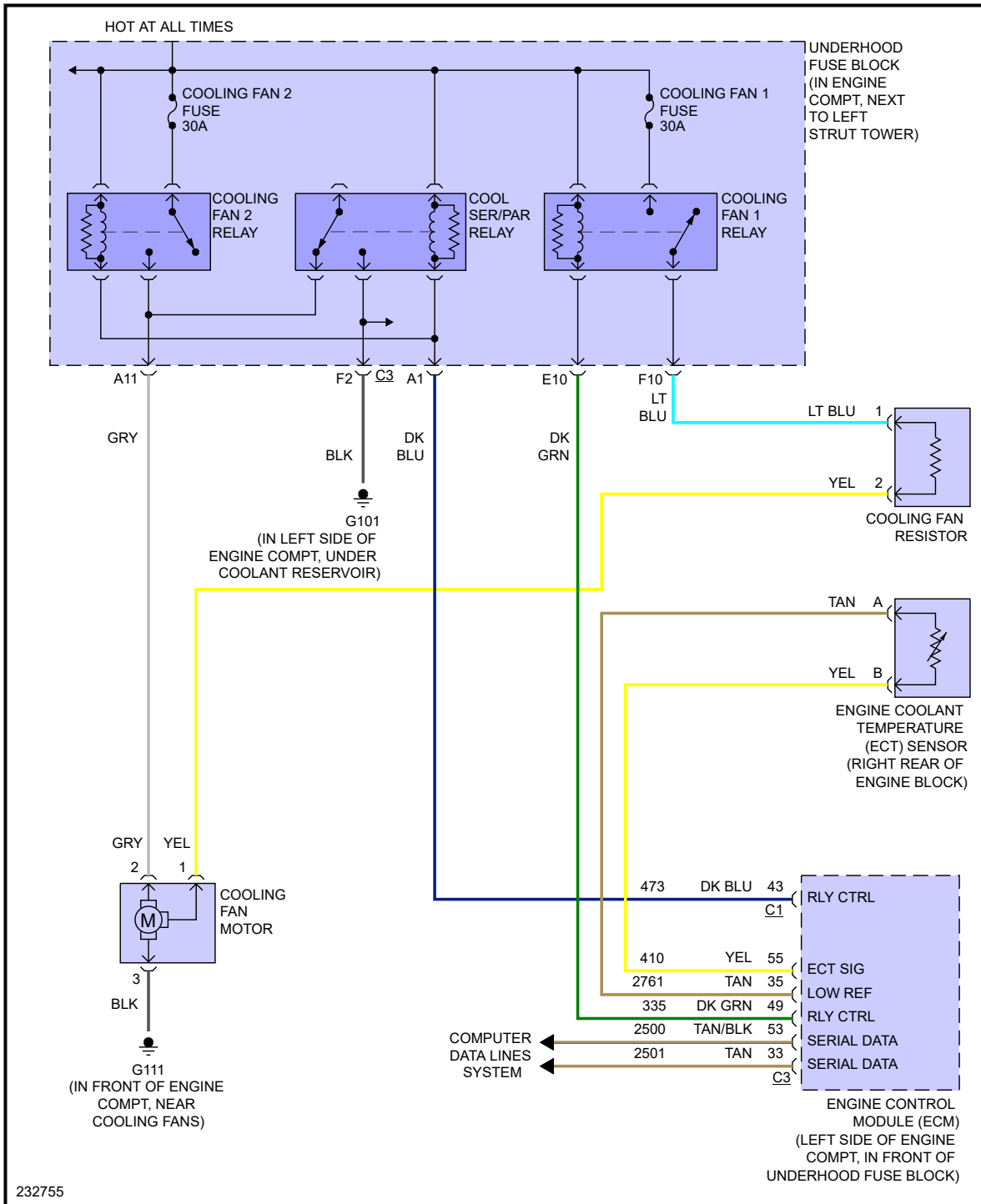
Fig 1: 2.4L VIN B, Cooling Fan Circuit
