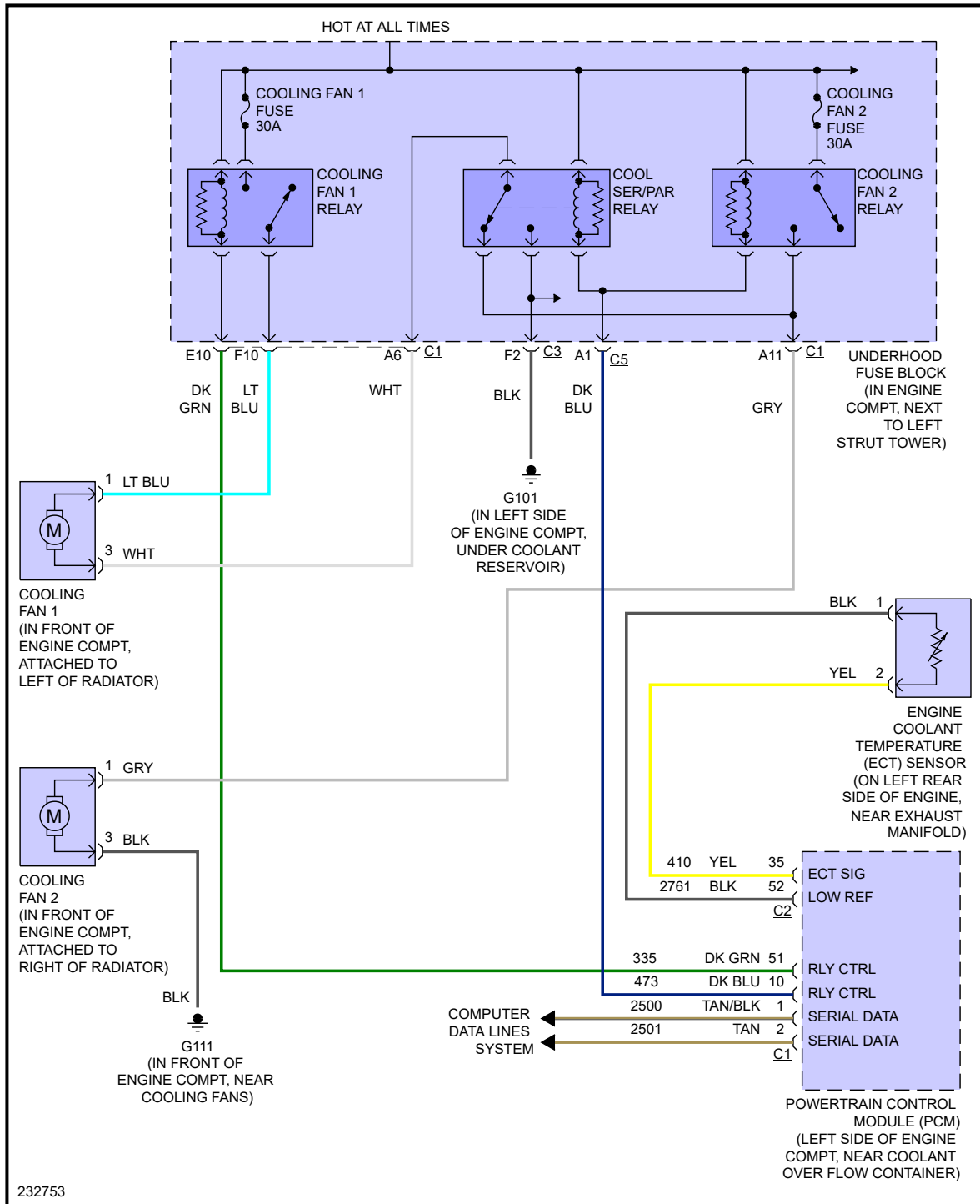
Fig 1: 2.0L VIN P, Cooling Fan Circuit
